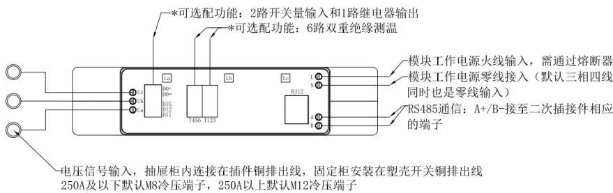
LQZ-35C\55C\51C接线图
